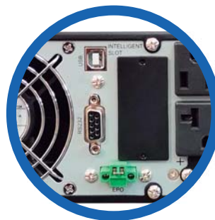
Puertos de comunicación y EPO
